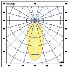
9D - 50°
