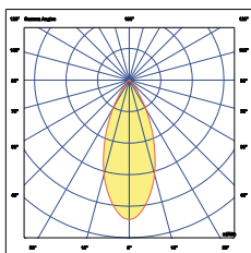
9C - 42°
