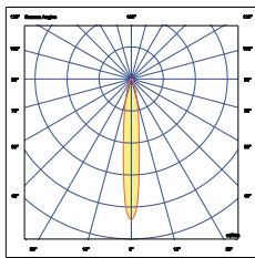
9A - 12°
