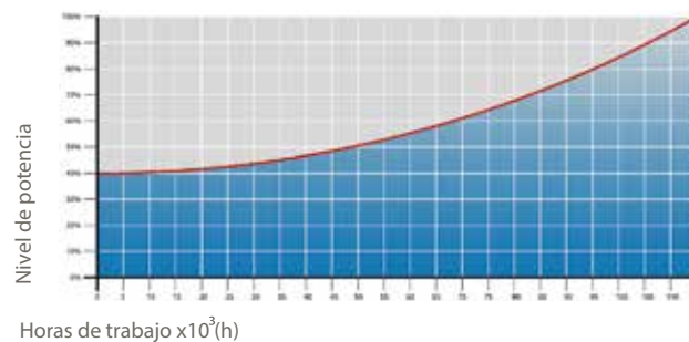
CLO | Compensación del flujo luminoso
