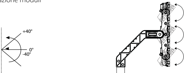
Rotazione moduli
