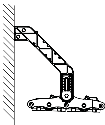
Installazione a parete
