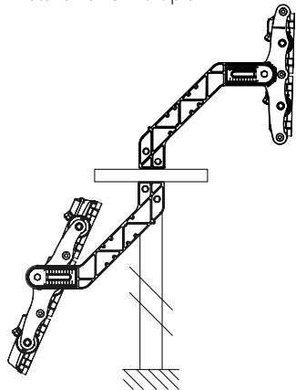
Installazione multipla
